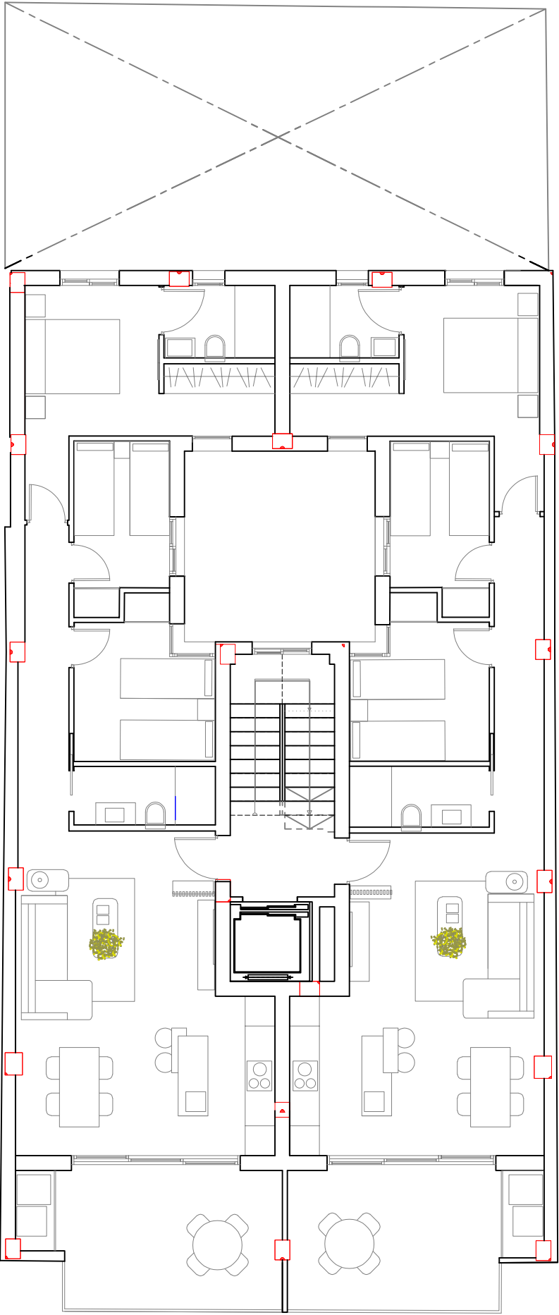
PLANTA 1-2-3
